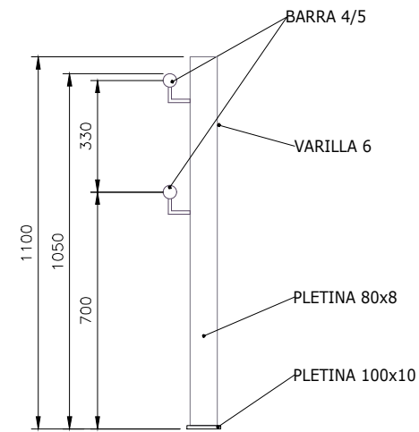
DETALLE BARANDILLA DOBLE PASAMANOS Escala: 1/20
