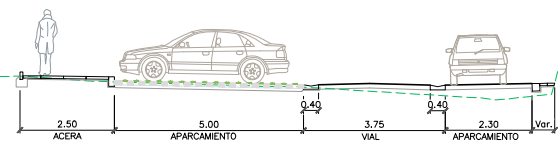
SECCION 8-8
