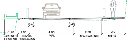
SECCION 15-15
