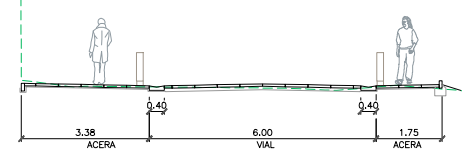
SECCION 10-10
