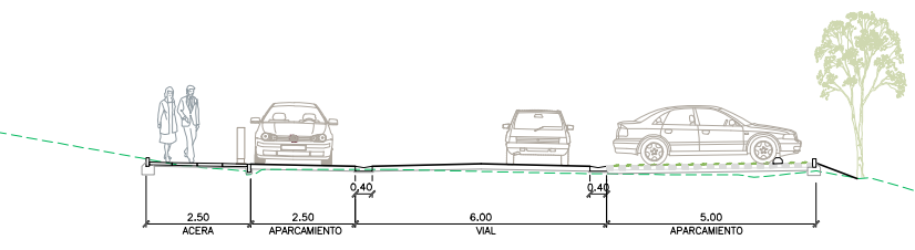
SECCION 12-12
