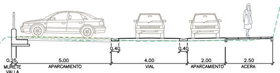
SECCION 16-16
