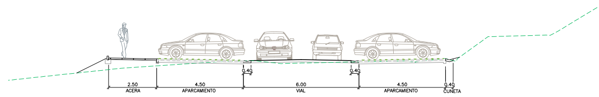
SECCION 13-13
