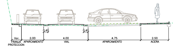
SECCION 18-18
