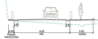
SECCION 19-19
