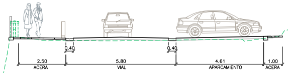
SECCION 9-9
