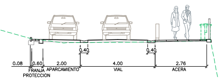
SECCION 17-17
