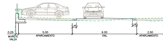
SECCION 7-7
