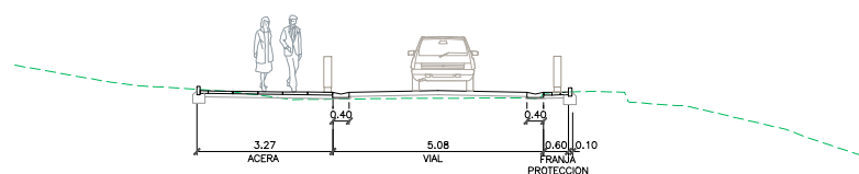
SECCION 4-4
