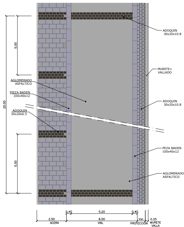
SECCION 2-2
