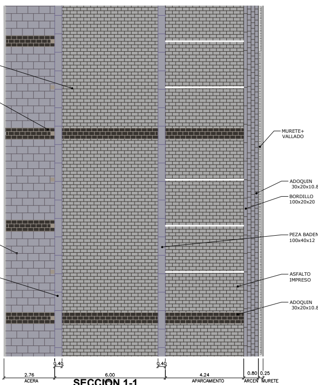
SECCION 1-1
