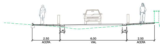
SECCION 6-6
