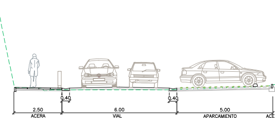
SECCION 4-4
